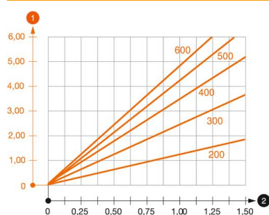
Диаграма на натоварване конзола тип AS 15
