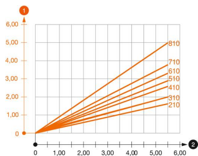
Диаграма на натоварване конзола тип AS 55
